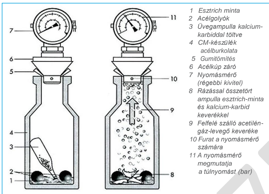
4. ábra - CM-készülék A vizsgált minta maradék nedvességtartalmának meghatározása. [MÉVSZ Kerámiaburkolatok kialakításának műszaki irányelve]
