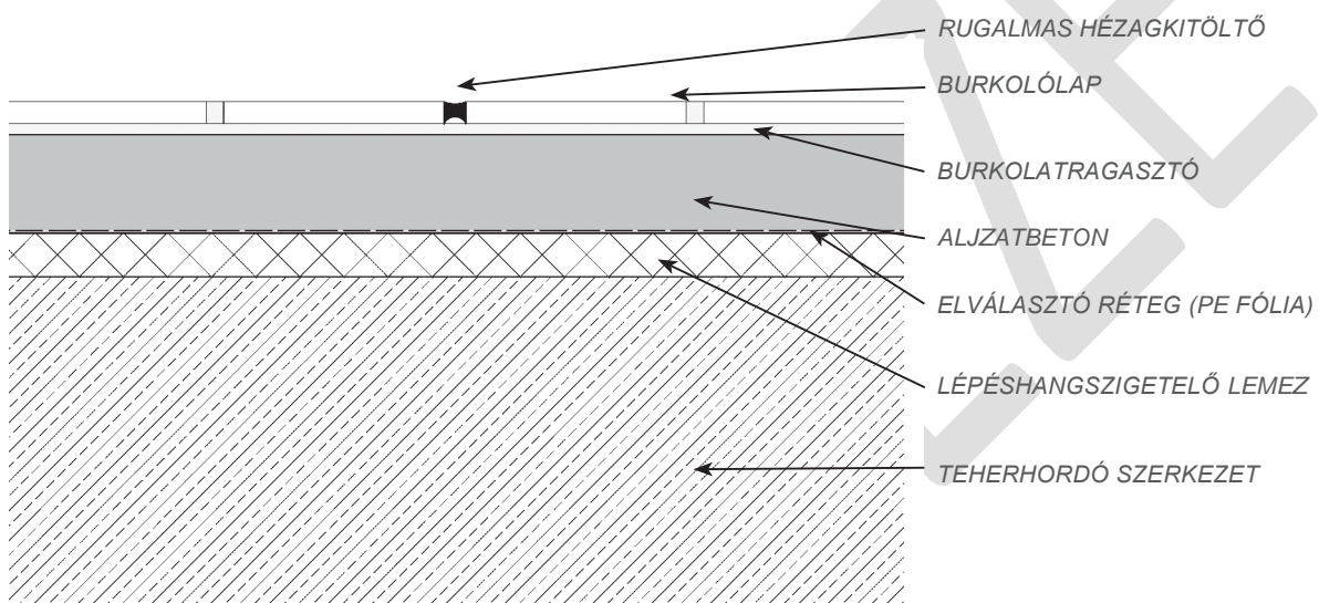
9. ábra – Burkolatdilatáció vázlata [MÉVSZ Kerámiaburkolatok kialakításának műszaki irányelve]
