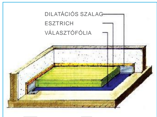
csúsztatott esztrich
