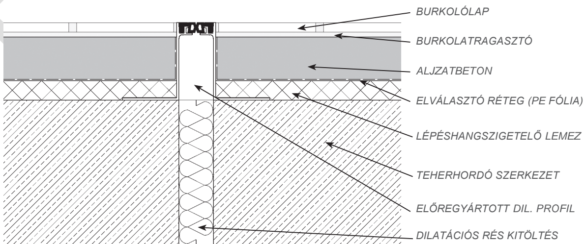
7. ábra – Szerkezeti dilatáció vázlat
