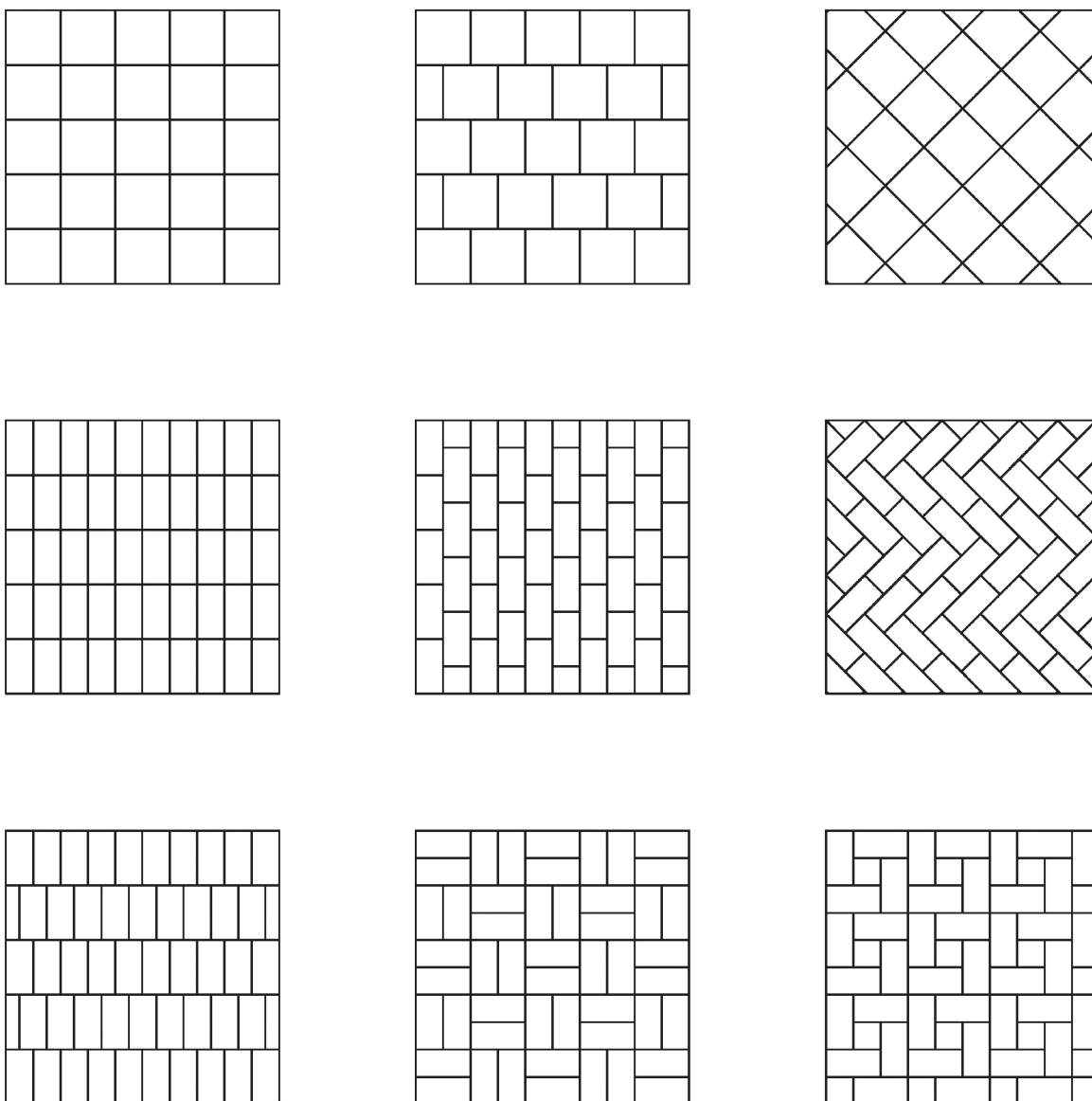
1. ábra Jellemző burkolatkialakítások [MÉVSZ Kerámiaburkolatok kialakításának műszaki irányelve]
