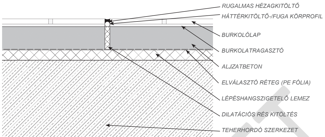
8. ábra – Aljzatdilatáció vázlata [MÉVSZ Kerámiaburkolatok kialakításának műszaki irányelve]
