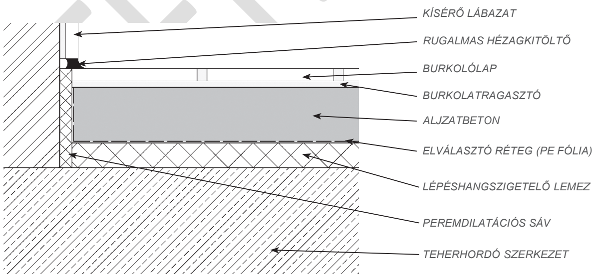
10. ábra – Peremdilatáció vázlata [MÉVSZ Kerámiaburkolatok kialakításának műszaki irányelve]
