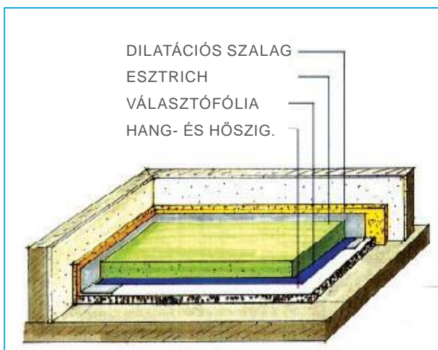
úsztatott esztrich
