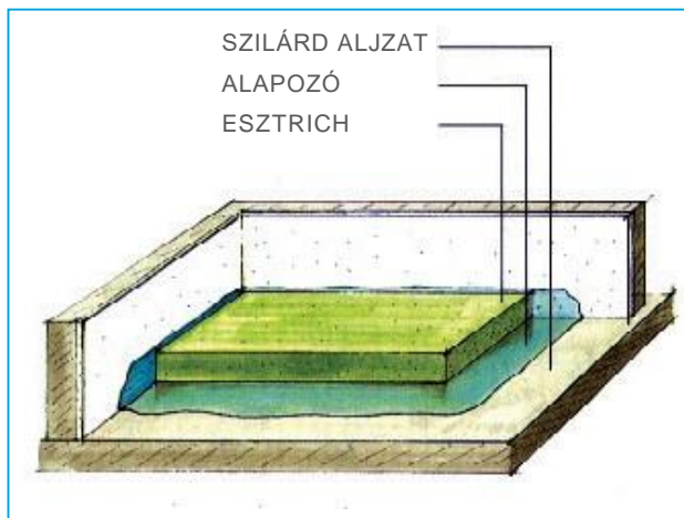
kötött esztrich
