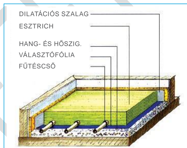
hűtött/fűtött esztrich
