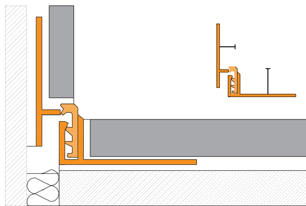
13. ábra – Előregyártott peremdilatációs profil vázlata [MÉVSZ Kerámiaburkolatok kialakításának műszaki irányelve]
