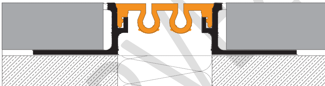
11. ábra – Előregyártott szerkezeti dilatációs profil vázlata [MÉVSZ Kerámiaburkolatok kialakításának műszaki irányelve]
